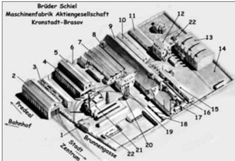
Ansicht der Fabrik um 1930 (nach einer isometrischen Zeichnung).
